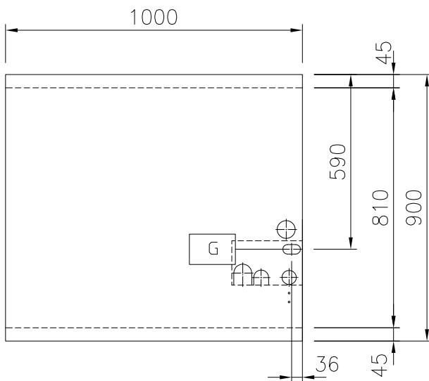
Boven aanzicht
